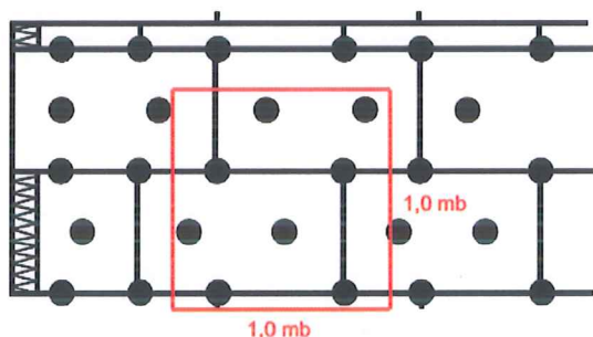
Schemat układu kołków w strefie przynaróżnikowej -8 sztuk /m 2
