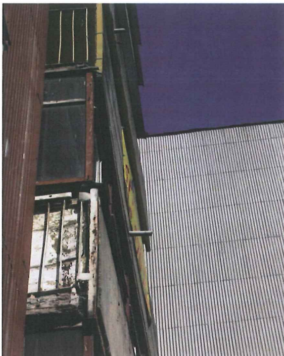
Fot.1. Widok na fragment elewacji z loggiami - średni -zły stan techniczny większości balustrad loggii.
